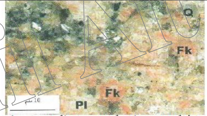
الوثيقة (10): صورة لعينة الغرانيت ملاحظة بالعين المجردة
