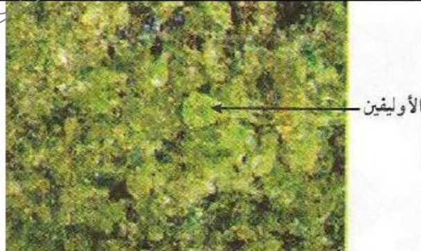
الوثيقة (14): صورة لعينة البيريدوتيت ملاحظة بالعين المجردة
