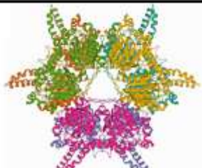
الوثيقة 2 البنية الفراغية لانزيم MCC3
