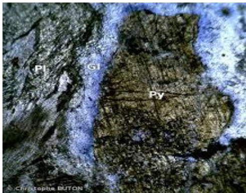
ميتاغابرو ذو غلوكونان سحنة الشبيست الأزرق
