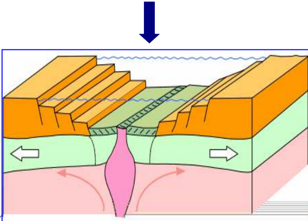
3 بداية تشكل ريفت اللوح المحيطي
