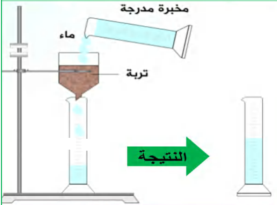
تجربة توضح خاصية النفاذية في التربة
