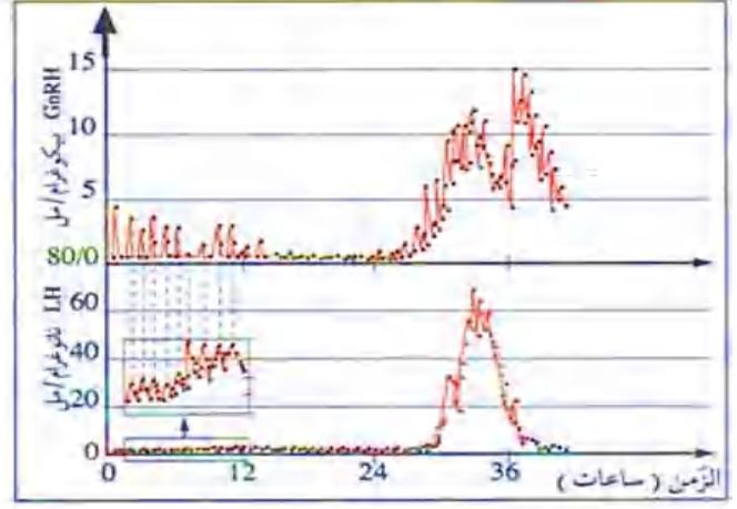
الوثيقة 7 : معايير توضيح إفراز LH و GnRH (عند تعجئة في نهاية المرحلة الجريبية)
