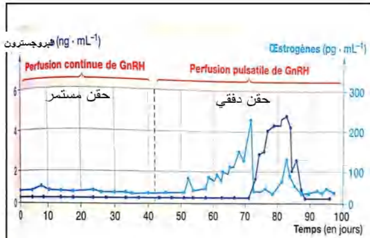
وثيقة 8: تأثير الحقن المستمر والدفعي لهرمون GnRH على الهرمونات المبيضية
