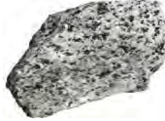
الغرانيت صخر ناري ( ماغماتي ) يتصلب ببطء تحت سطح الأرض
