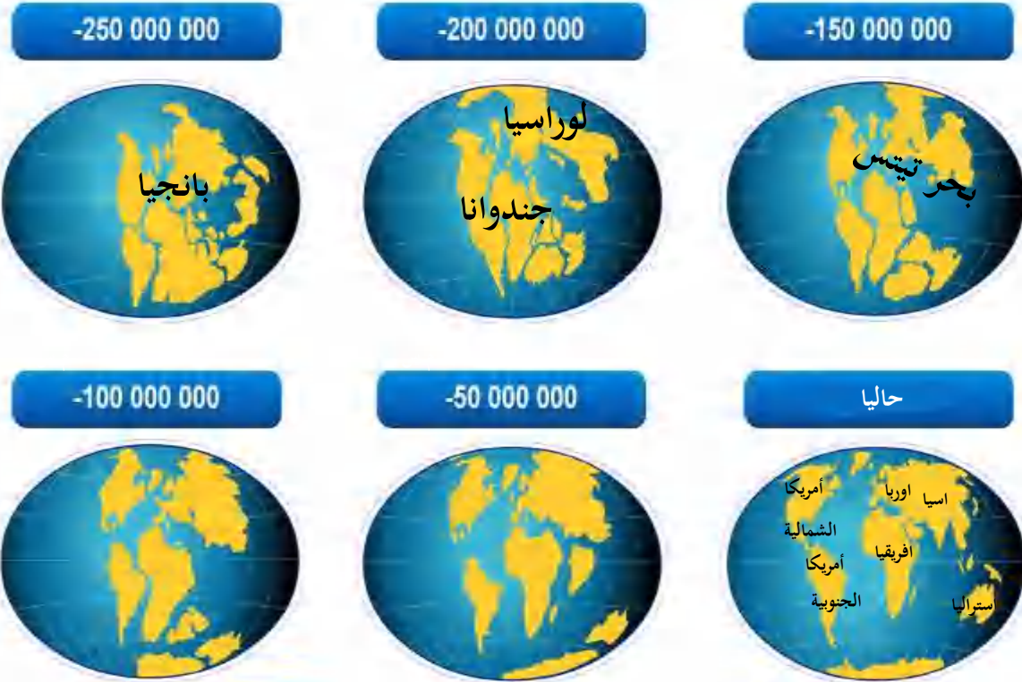
السند الأول : مراحل زحزة القارات حسب نظرية فيجنر
