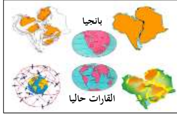
الوثيقة 01: شواهد العالم
