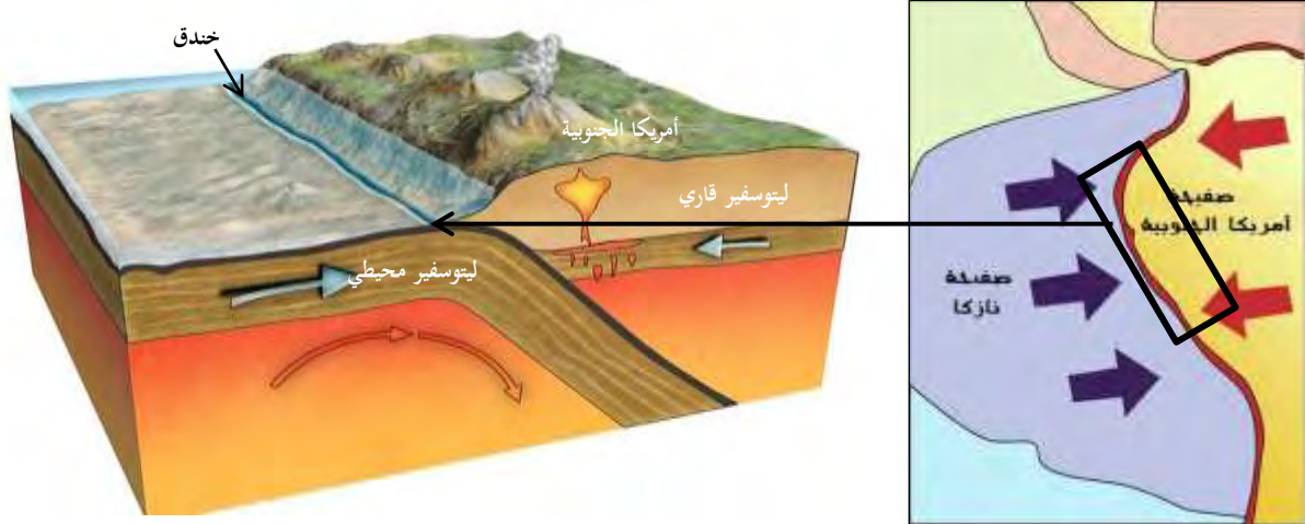
السند الأول : تقارب الصفائح
